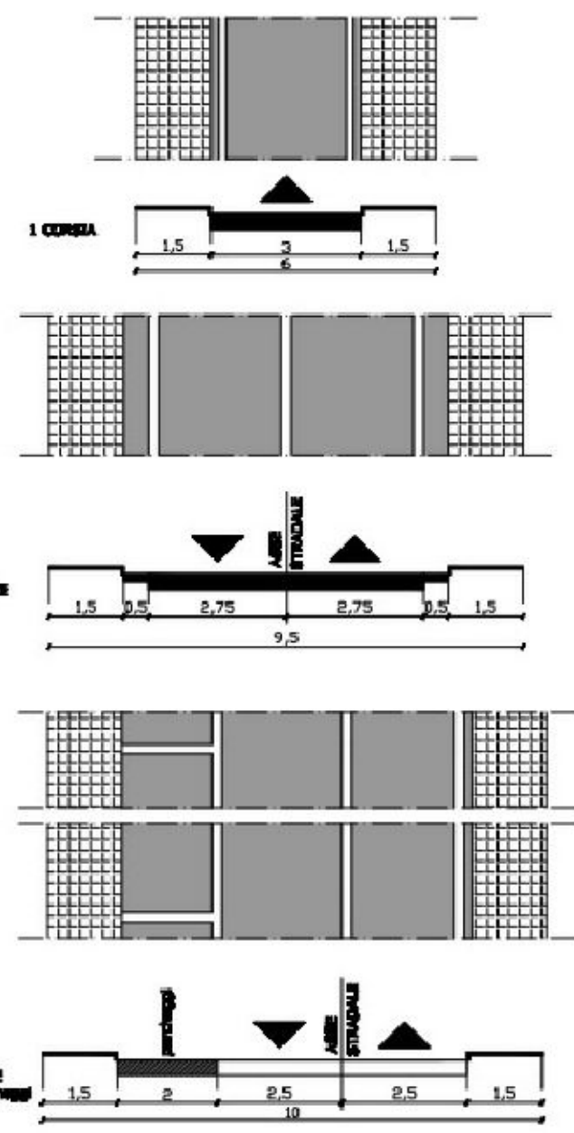
STRADE LOCALI AMBITO URBANO scala 1:100
